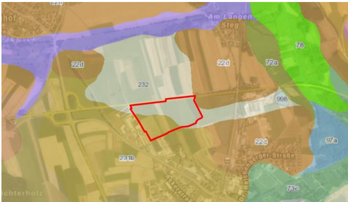
Abbildung 9: Ausschnitt Übersichtsbodenkarte 1:25.000
